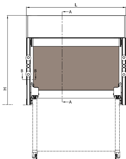
guida a parete - wall guide
