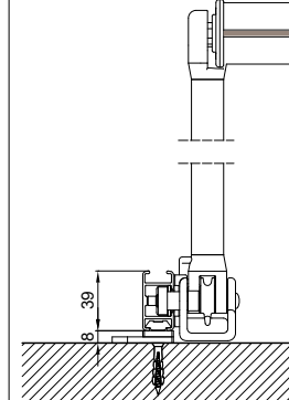
guida a nicchia - niche guide B-B
