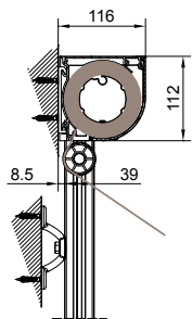
TONDO - ROUND A-A
