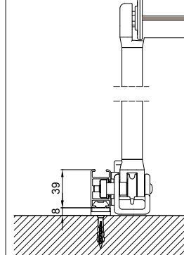
guida a parete - wall guide B-B
