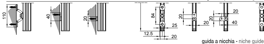
guida a parete - wall guide
