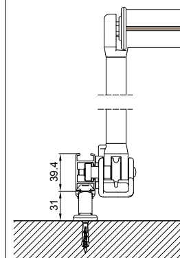
guida a parete - wall guide B-B
