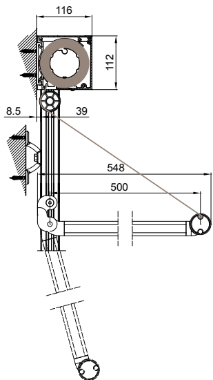
guida a parete - wall guide
