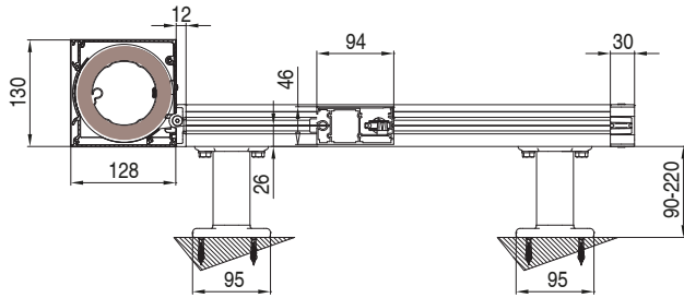
supporto guida regolabile - Adjustable guide support
