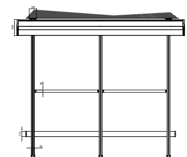
Vista dall'alto (3 profili guida) Top view (3 guide profiles)
